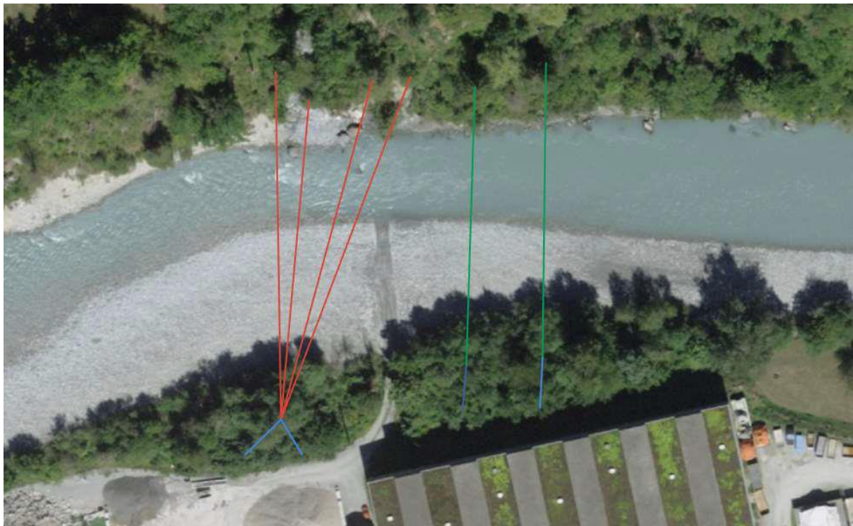
Abbildung: Skizze für mögliche Standorte der Tragseile. Rot permanente Seile, grün demontierbare Seile, blau Abspannseile
